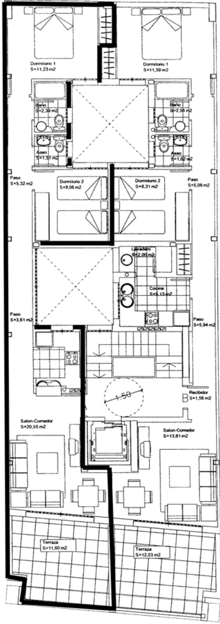
PLANTA ATICO
