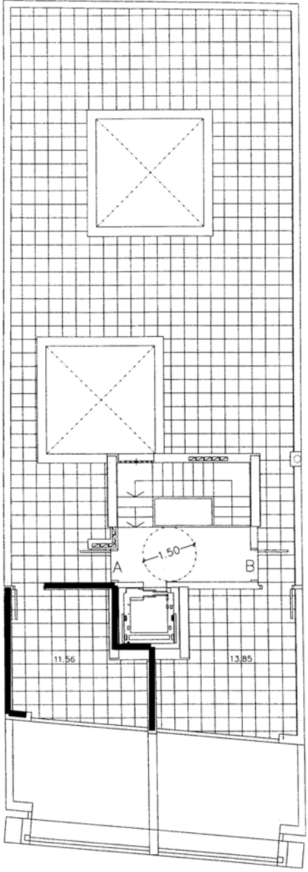
CUBIERTA
